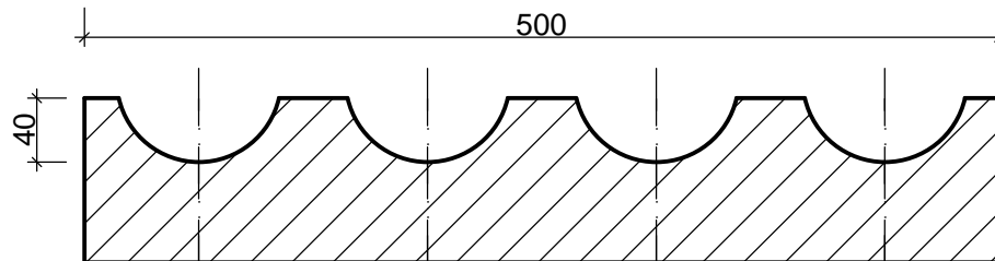
przekrój A-A
