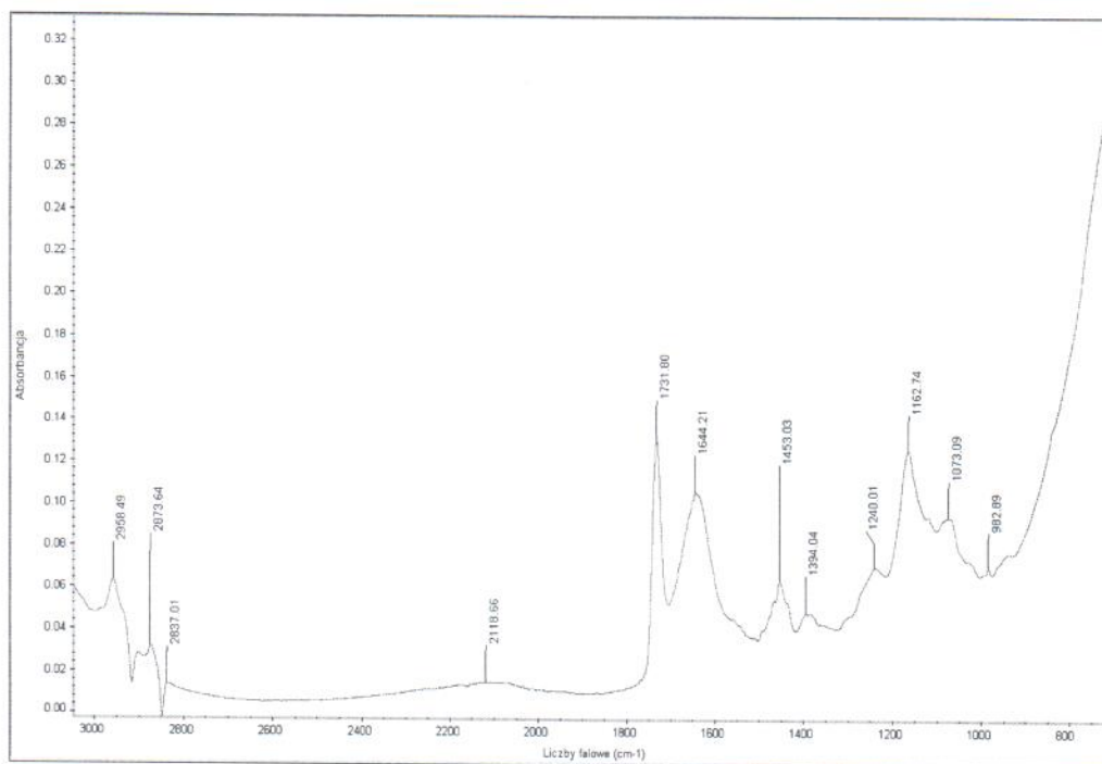
Rysunek 2 – Widmo w podczerwieni (analiza FTIR) materiału Murfill
